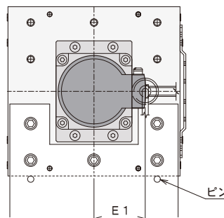
＜本体取付例 (X6305FWS)＞ ※4
