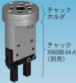
取付例
